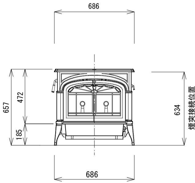
立面図
