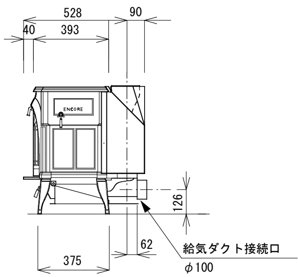
側面図
